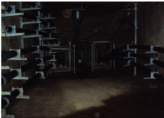
N0.11 신광명-천왕 #6
